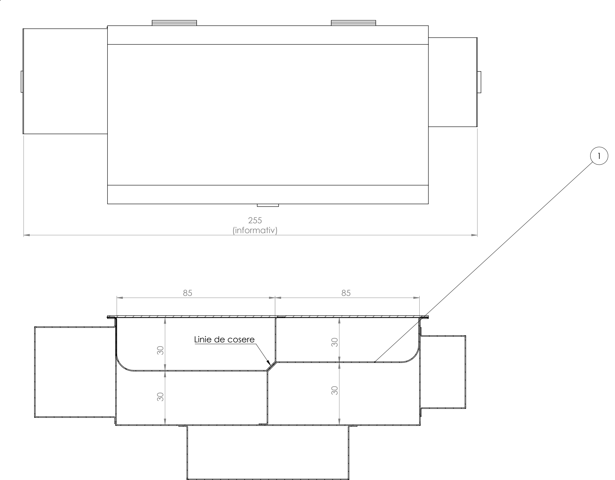
SECTIUNEA A-A
